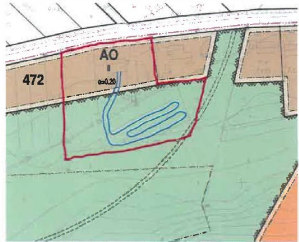
Kuva 9. Maalämpöjärjestelmän keräysputkiston likimääräinen sijainti kaavakartalle sijoitettuna. Punaisella esitetty aluerajaus on minimi AO-korttelialueen rajaus, jolle putket mahtuvat.
