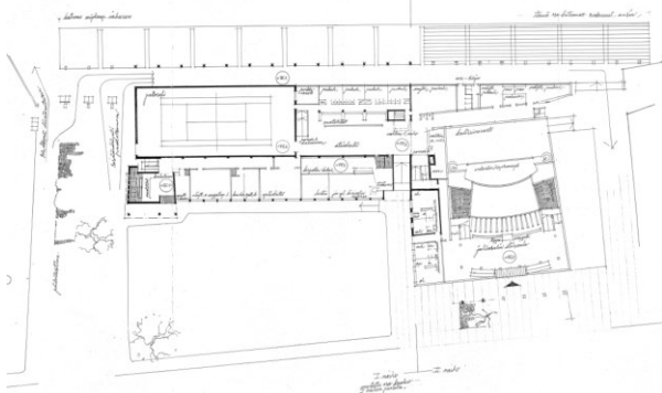
Kuva 16. Kouvolan sivistys- ja urheilutalo, maantasokerros, arkkitehti Eero A. Kajava, alustava luonnos 23.2.1952.
