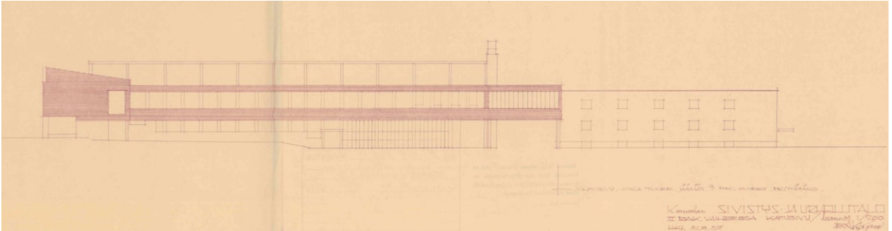
Kuva 21. Kouvolan sivistys- ja urheilutalo, 2. vaihe / eteläjulkisivu. Arkkitehti Eero A. Kajava 5.3.1956. Tiilirakenteinen toimisto-osa sijoittui kuntotalon itäpäättyyn siten, että rakennusten toiset kerrokset oli yhdistetty käytävällä toisiinsa. Toisessa vaiheessa myös laajennettiin pesäpallokentän puolella olevaa katosta sen nykyiseen laajuuteen.
