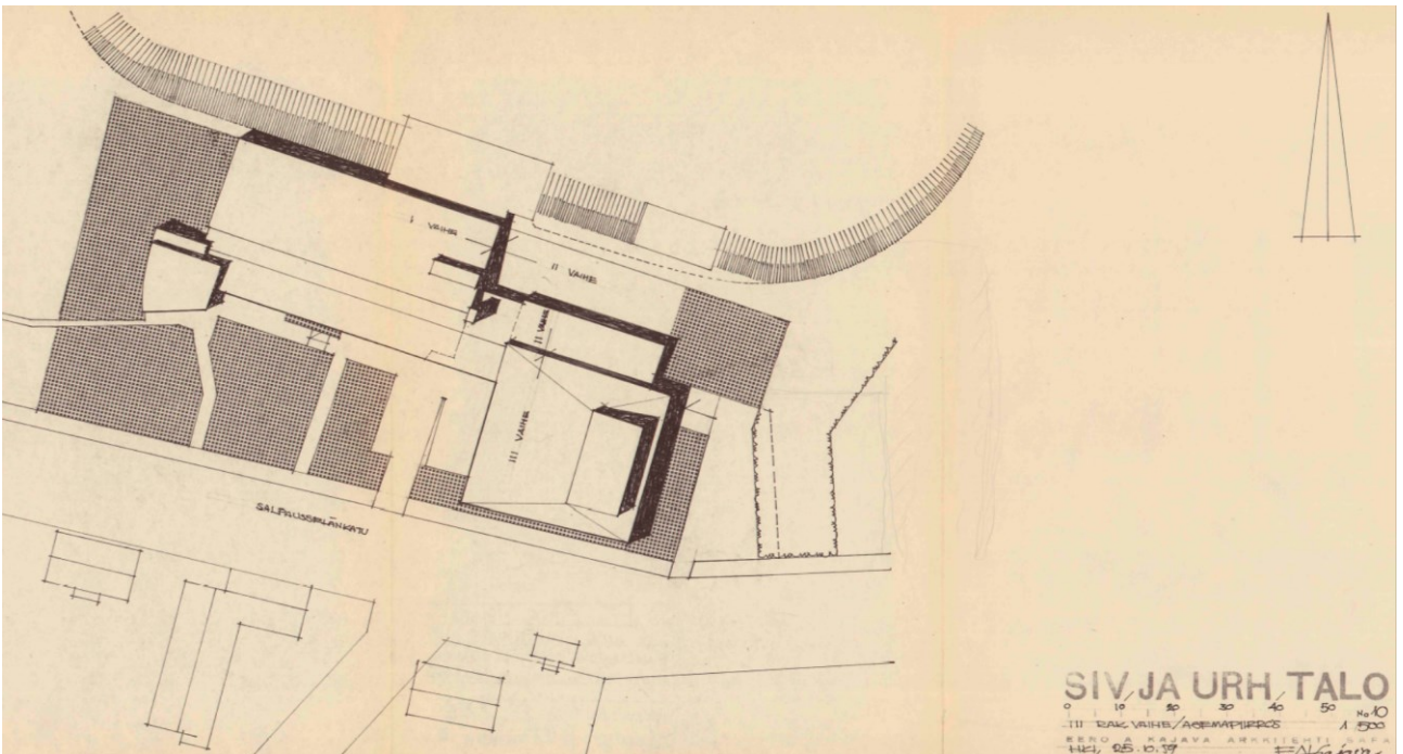
Kuva 24. Kouvolan sivistys- ja urheilutalo, 3. vaihe / teatteri, asemapiirros (rakennuslupa). Arkkitehti Eero A. Kajava 25.10.1959. Oheisestä asemapiirustuksesta puuttuu katsomon 2. vaiheen laajennus. Huomioitavaa on se, että kuvassa olevaa teatterirakennusta on laajennettu kuvassa oikean suuntaan vuonna 1986 valmistuneessa peruskorjauksessa. Samassa yhteydessä on muutettu rakennuksen piha-alueita.
