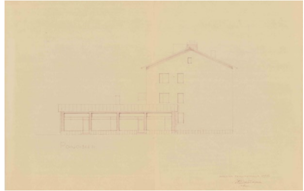
Kuva 75. Rakennuksen pohjoisjulkisivu.
