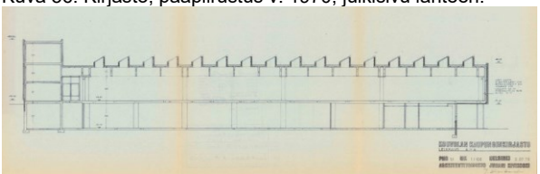
Kuva 57. Kirjasto, pääpiirustus v. 1970, leikkaus A-A.
