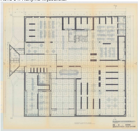
Kuva 55. Kirjasto, pääpiirustus v. 1970, 1. kerros.
